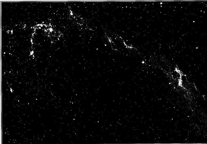
سديم البرقع في الدجاجة - المدعو أحياناً الطخور - حطام متجدد أعظم، التقطت هذه الصورة في مرصد بالومار، الشكل المقوس الذي لا يخلو من المفزى، يبعد عنّا (٢٥٠٠٠) سنة ضوئية. وقد حسب بالاستناد إلى حركات الغاز فيه، أن الانفجار المتجدد الأعظم قد حصل قبل (٥٠٠٠٠) سنة، وسيفقد ضياءه بعد (٢٥٠٠٠) سنة.
