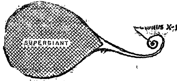
( شكل رقم ٥ - ٥ ) الثقب الأسود يتتبع نجما ضخما
