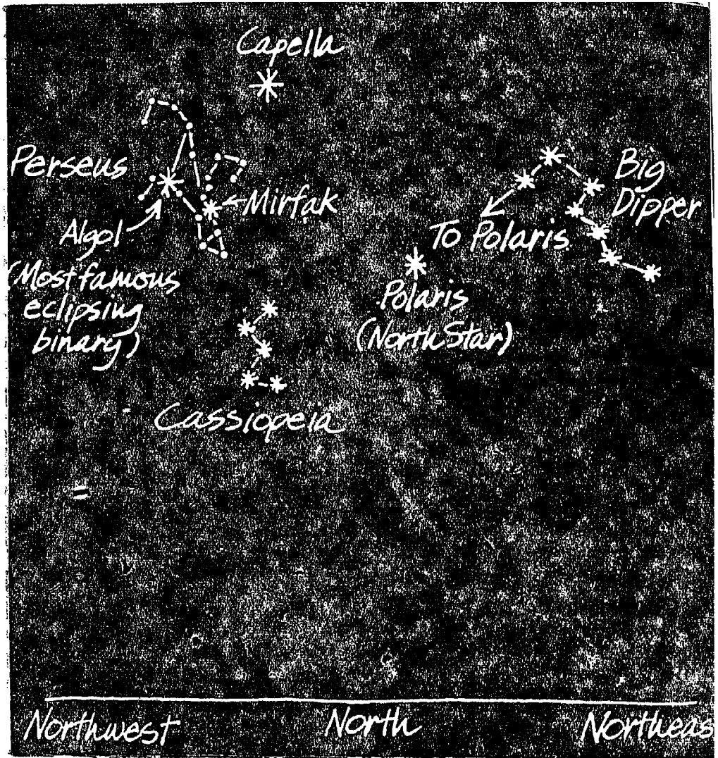
شكل ( ٦ - ١ ) : كيفية تحديد موقع النجم القطبي الشمالى ( بولاريس )
